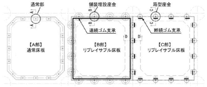
図-4 試験対象床版平面図
