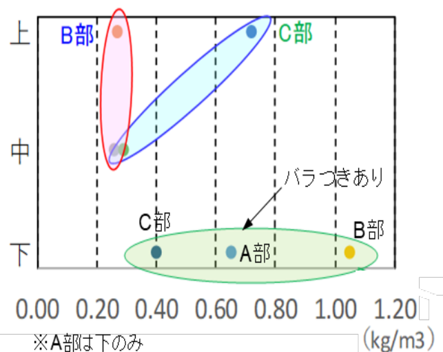
図-9 モルタルパネル試験結果分布図
