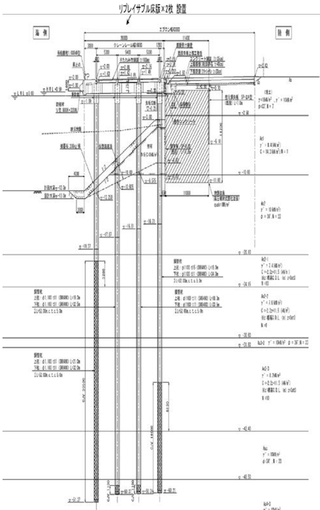
図-3 標準断面図 (リプレイサブル床版設置部)
