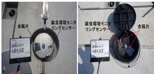
写真-3 座金内計測機器設置状況 （左：舗装埋設型座金（B部），右：箱型座金（C部））
