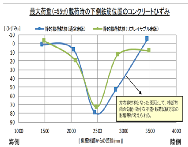
図-7 静的載荷試験結果
