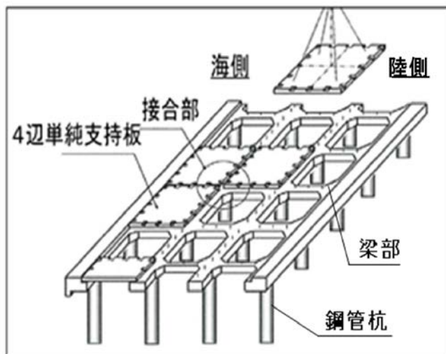
図-1 リプレイサブル棧橋イメージ図
