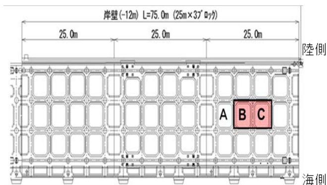
図-2 リプレイサブル床版（B・C床版）設置箇所
