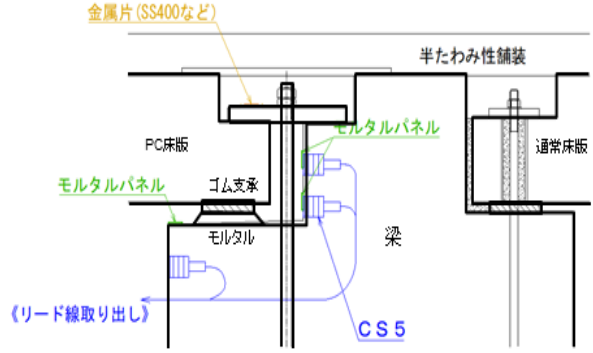
図-5 B-B断面図 (B部：舗装埋設型座金)
