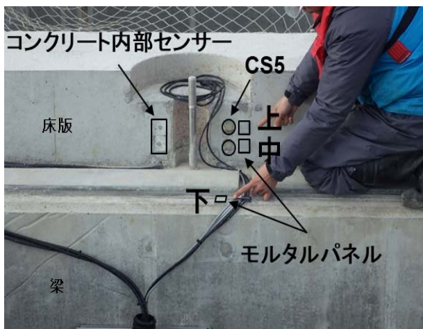
写真-4 梁内部計測機器設置状況
