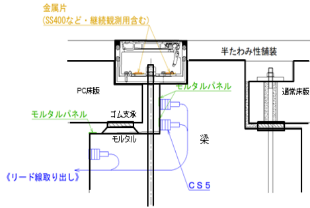
図-6 C-C断面図 (C部：箱型座金)
