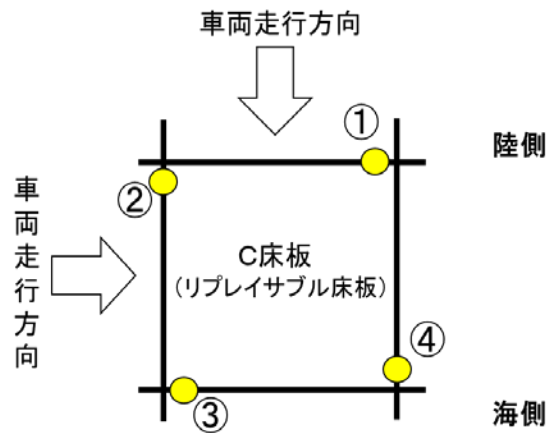
図-8 舗装目地幅計測箇所
