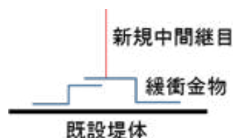
図-6 緩衝金物概要図
