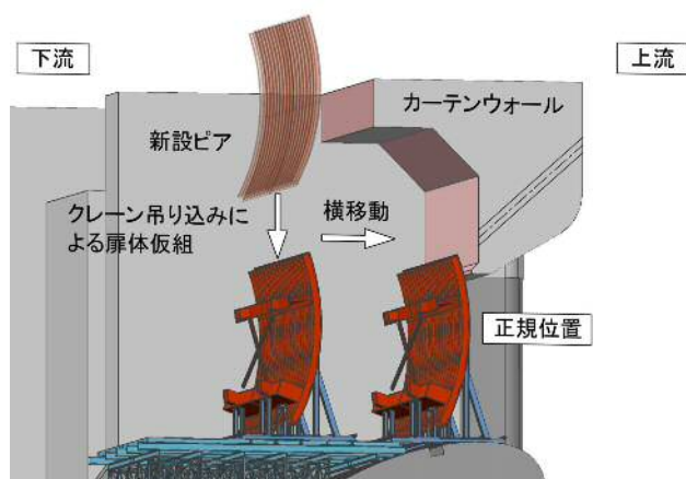
図-2 スライドインの概要図
