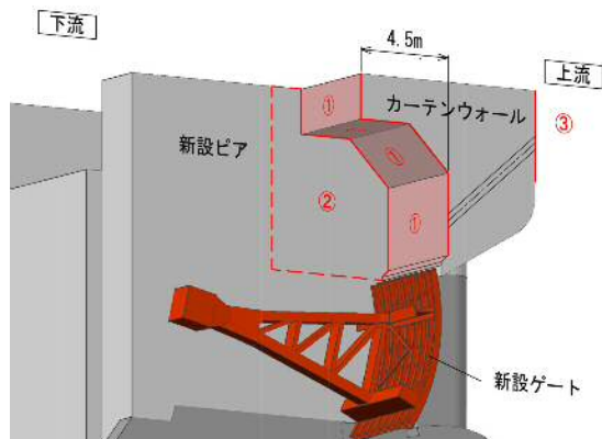
図-1 1号ゲートプレキャストの概要図
