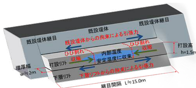
図-5 ひび割れ発生メカニズム
