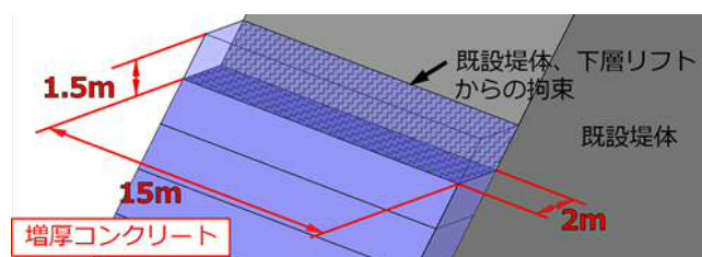
図-4 下流面増厚コンクリート概要図
